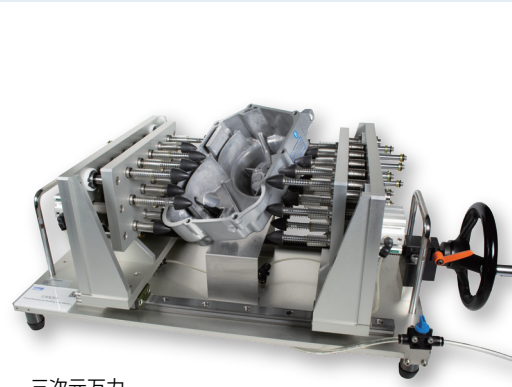
三次元万力
